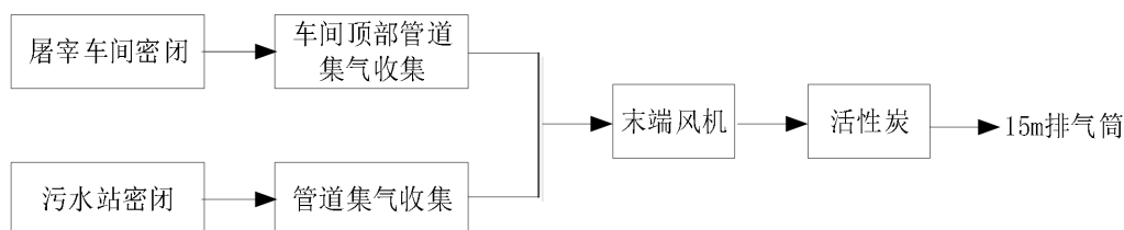
图 4-1 废气走向图
