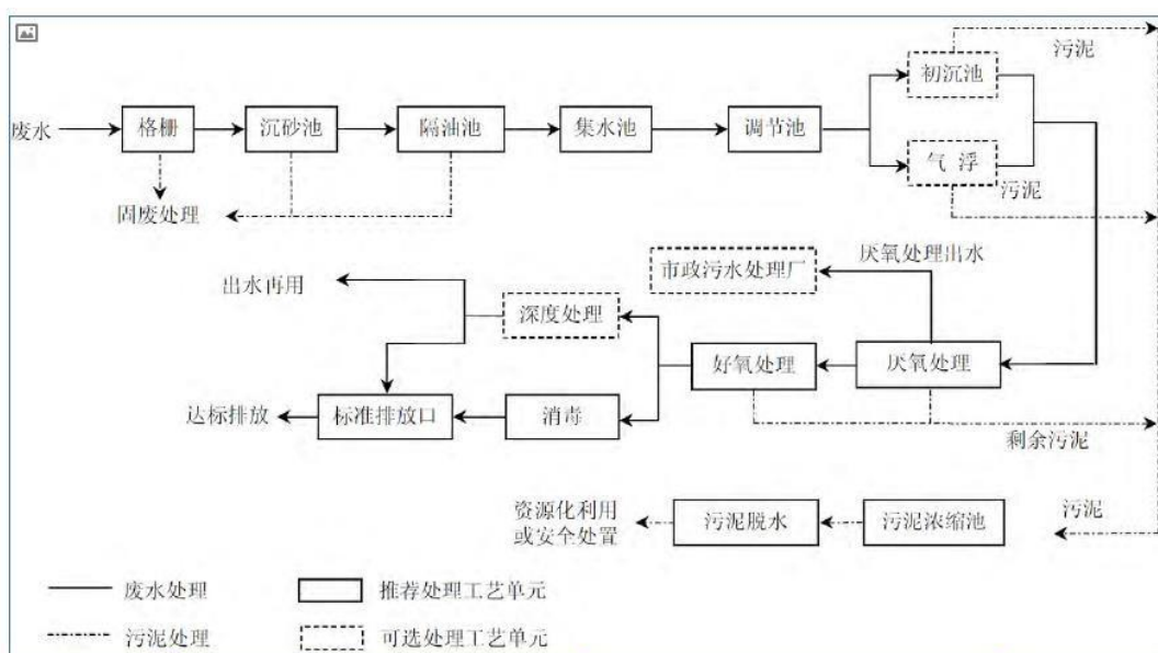
图 4-2 《屠宰与肉类加工废水治理工程技术规范》推荐及可选处理工艺
