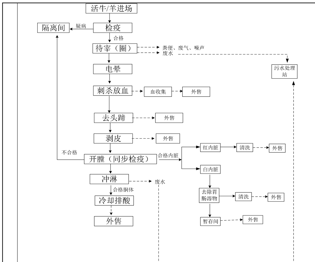
图 2-2 本项目屠宰工艺流程及产污节点图
