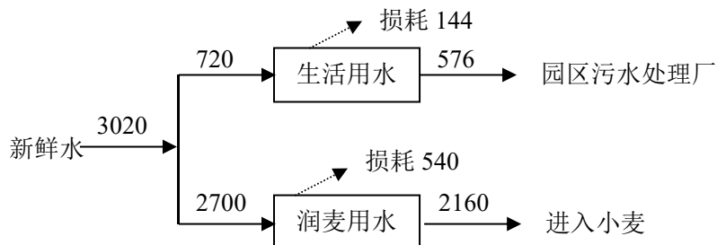
图 2-1 项目水平衡图 单位：m 3 /a
