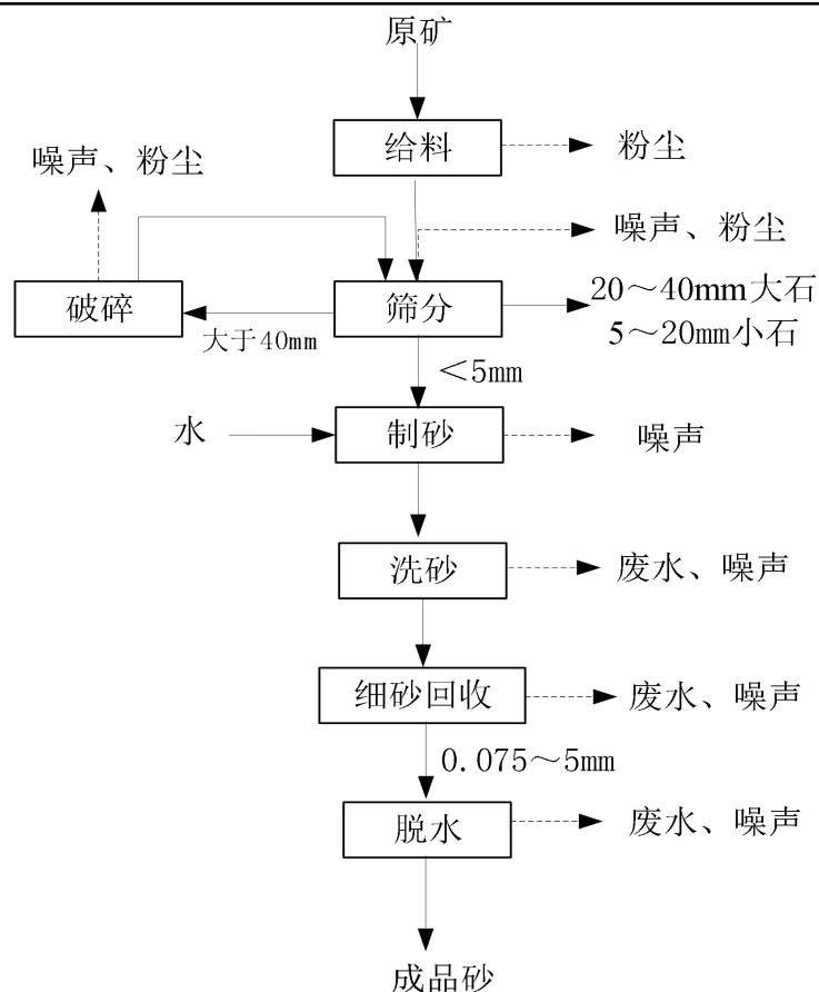
图 2-3 工业广场砂石加工工艺流程及排污节点图
