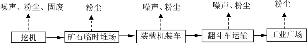
图 2-2 矿区开采工艺流程及排污节点图
