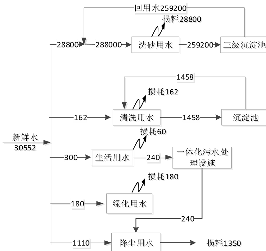
图 2-1 本项目水平衡图
