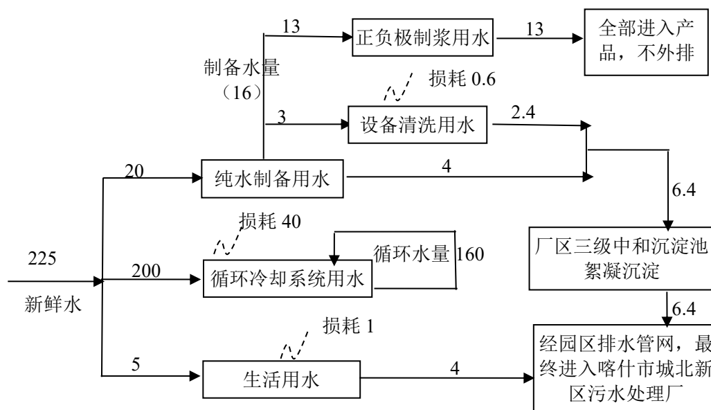
图 1 全厂用水量平衡图 (单位: \text{m}^3/\text{d} )
