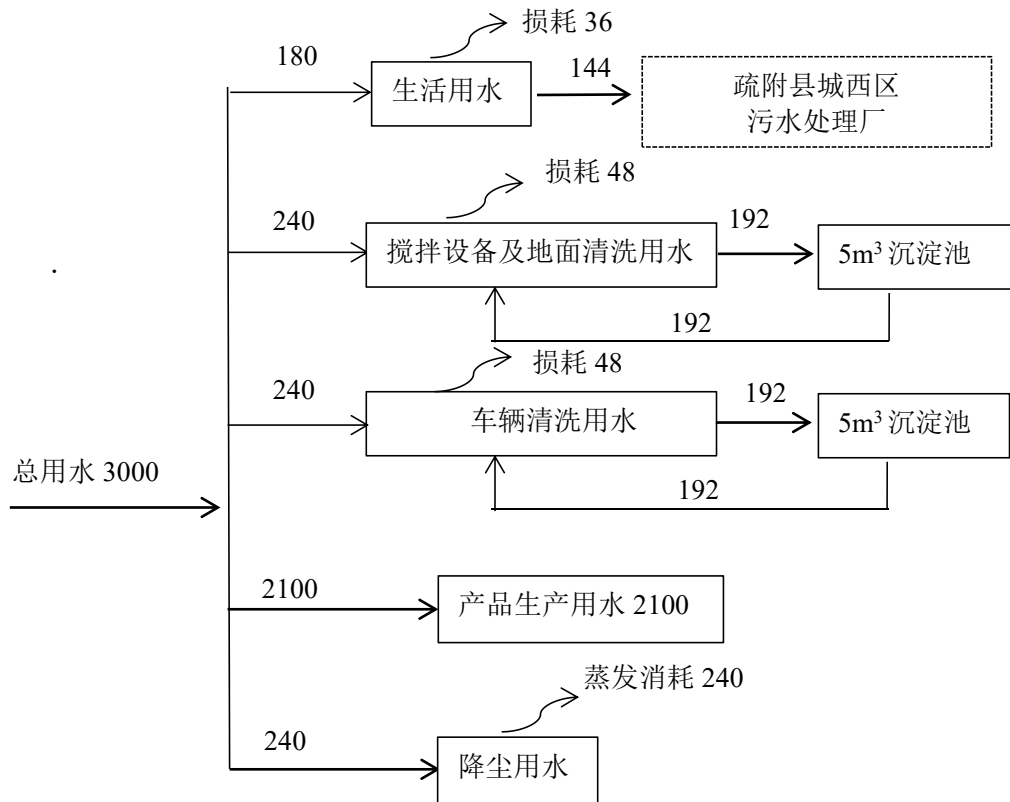
图 2-1 水平衡图 单位：m³/a
