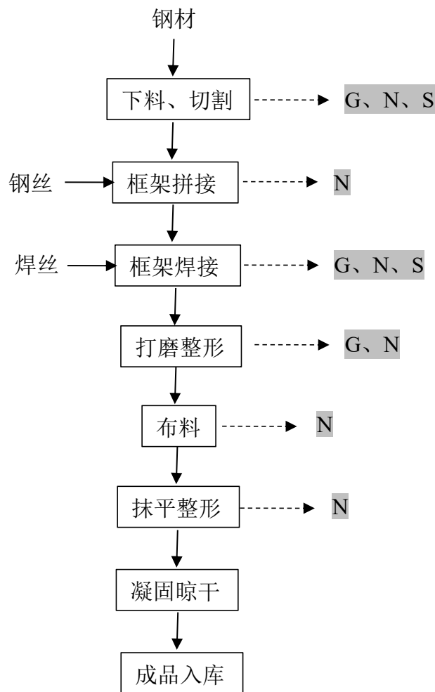
图 2-4 混凝土叠合板工艺流程及产污环节（G-废气、N-噪声、S-固废）
