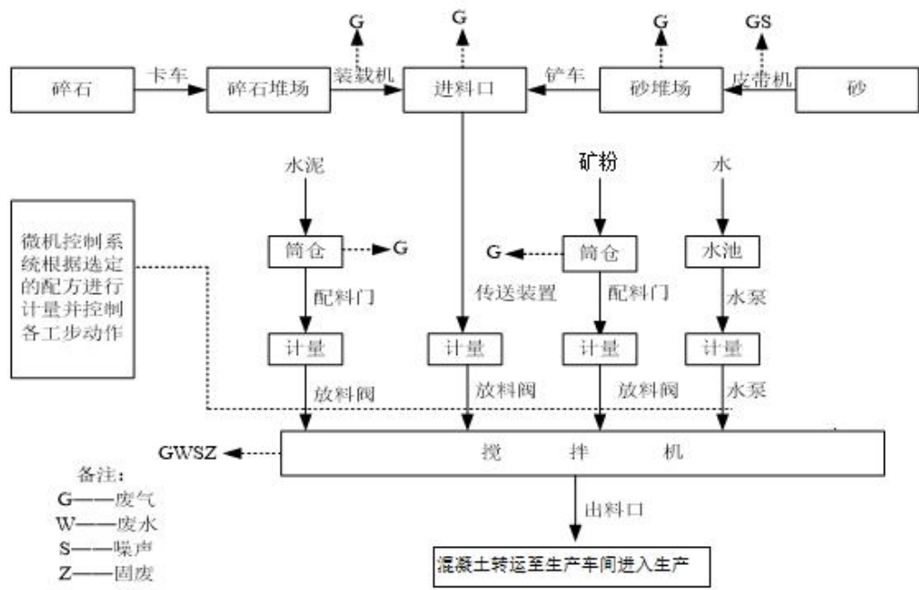
图 2-2 本项目混凝土工艺流程及产污节点示意图
