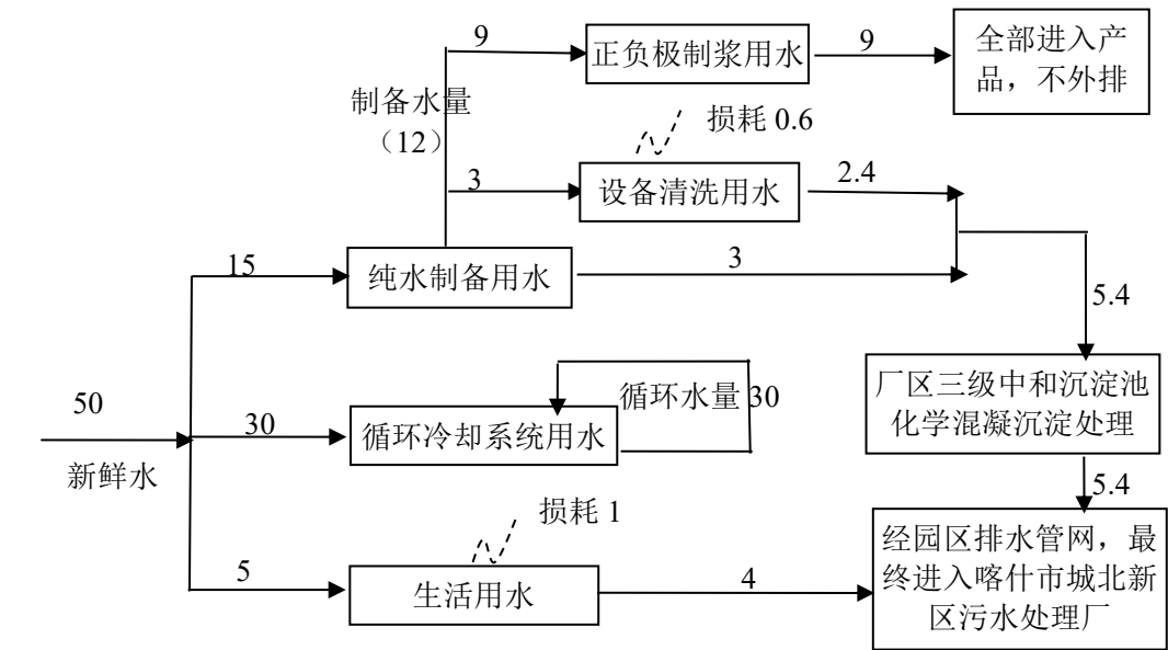
图 1 全厂用水量平衡图 （单位：m 3 /d）
