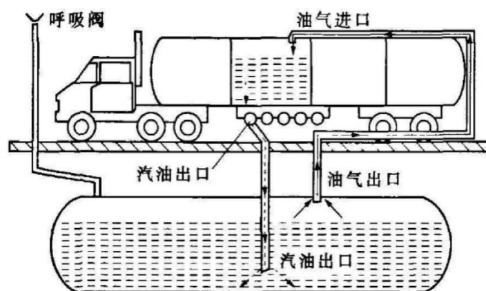
图2-2 卸油油气回收系统
