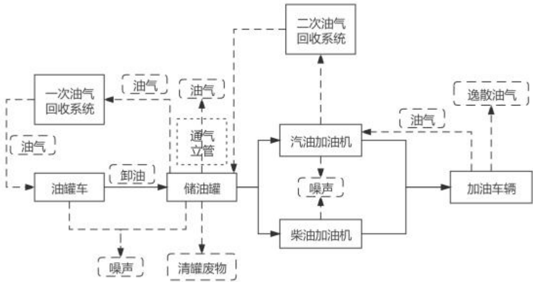
图2-1 卸油加油工艺流程及产污节点图
