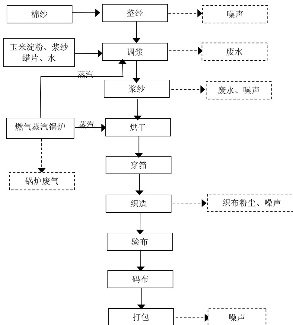
图3 项目运营期工艺流程及产污环节图
