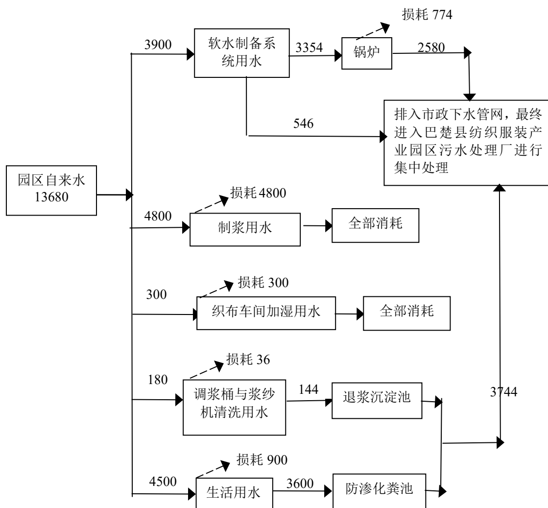
图1 水平衡图 （单位：m 3 /a）
