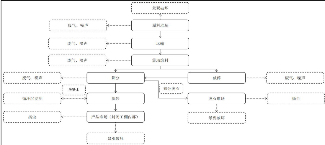
图 2-6 运营期矿石加工工艺流程及产污环节图
