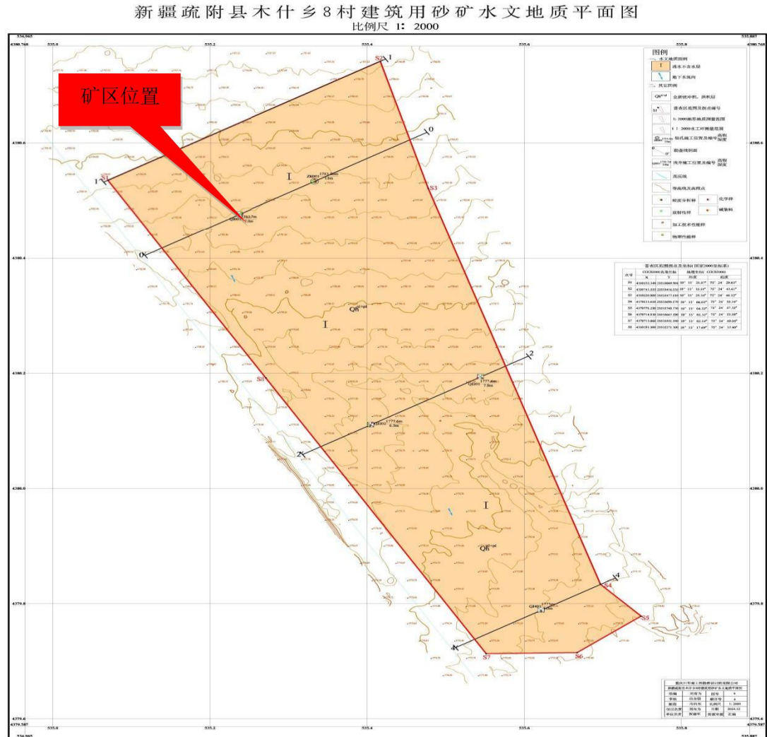
图 3-1 矿区水文地质图
