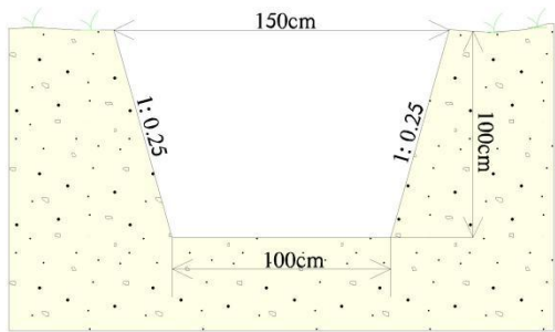
图 2-2 截水沟断面示意图
