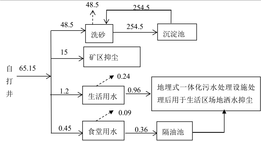
图 2-1 项目水量平衡示意图 (单位：m 3 /d)
