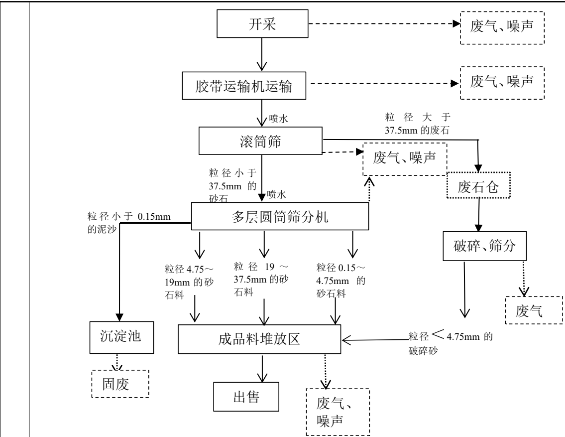
图 2-2 运营期工艺流程及其产污节点图
