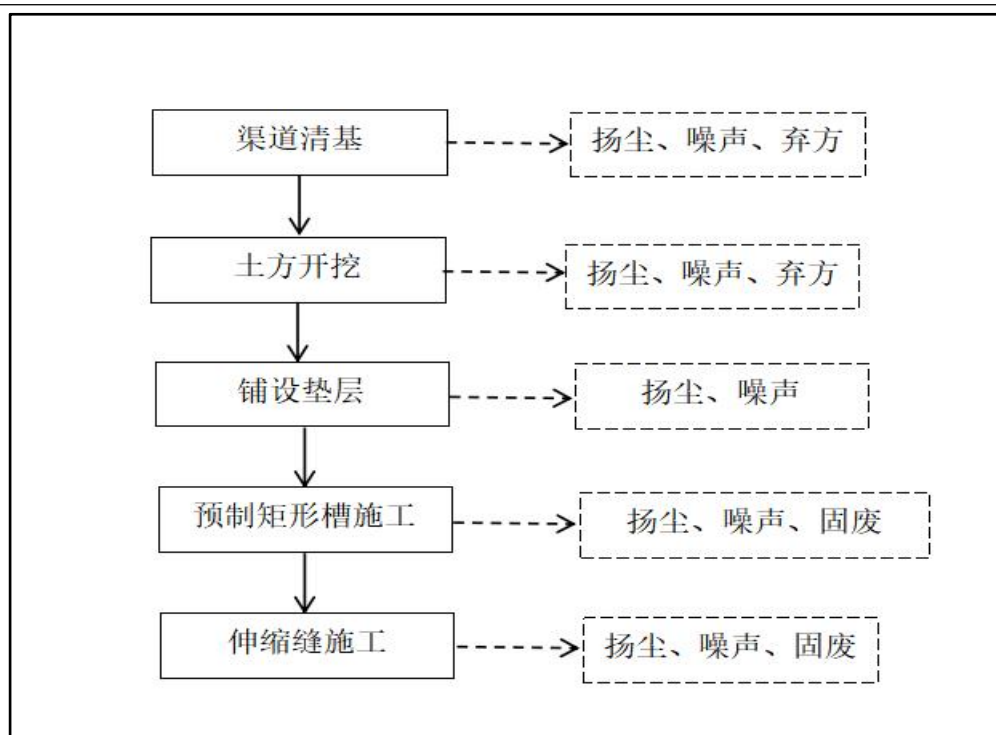
图 4 渠道施工期工艺及污染物产排流程图
