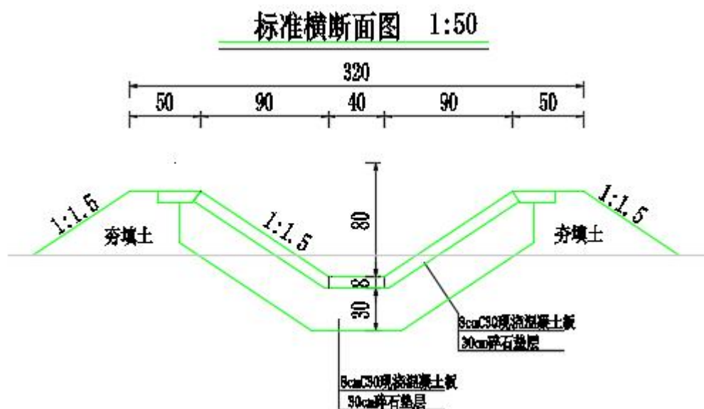
图 1 全断面现浇梯形断面设计图
