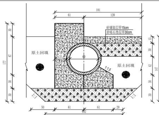
图 3 涵桥剖面示意图
