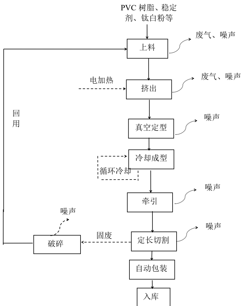
图 2.2-3 PVC 管生产线工艺流程及产污节点图
