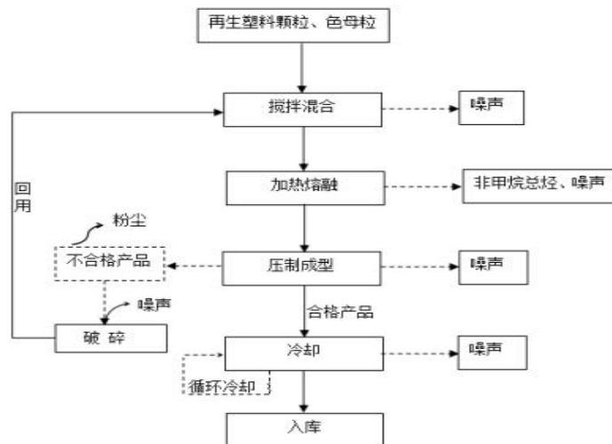
图 2.2-6 涂料桶生产线工艺流程及产污节点图
