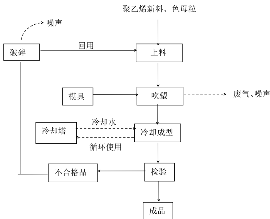
图 2.2-7 汽车玻璃水水瓶、水壶、洗衣液桶、水瓶 生产线工艺流程及产污节点图
