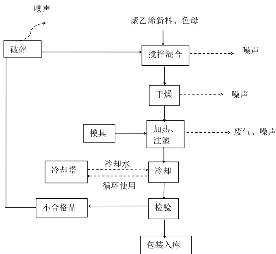
图 2.2-5 塑料日用品生产线工艺流程及产污节点图
