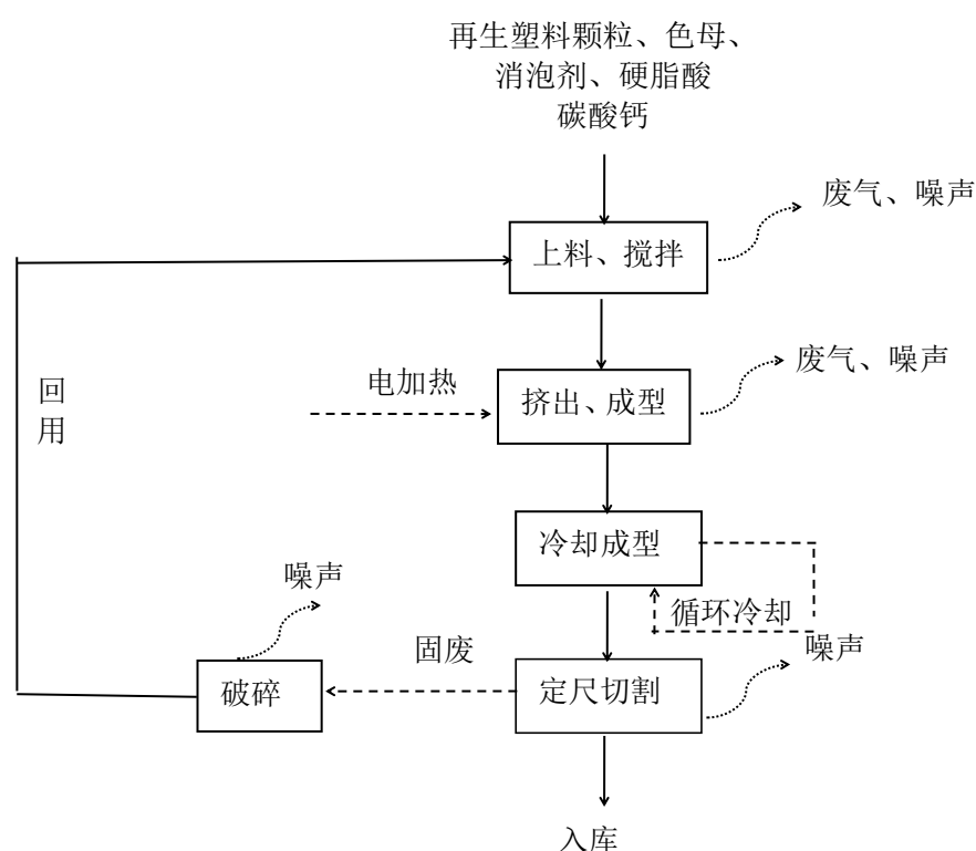
图 2.2-4 波纹管生产线工艺流程图
