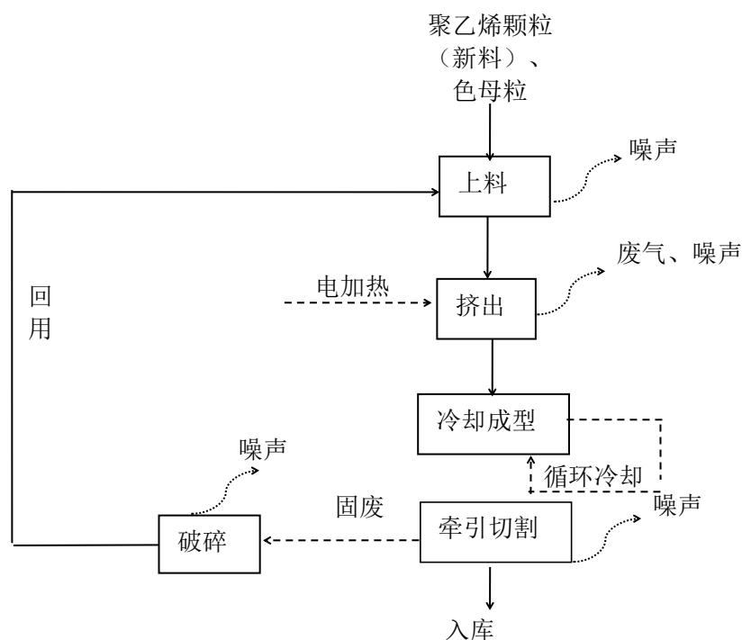
图 2.2-2 PE 给水管生产线工艺流程图
