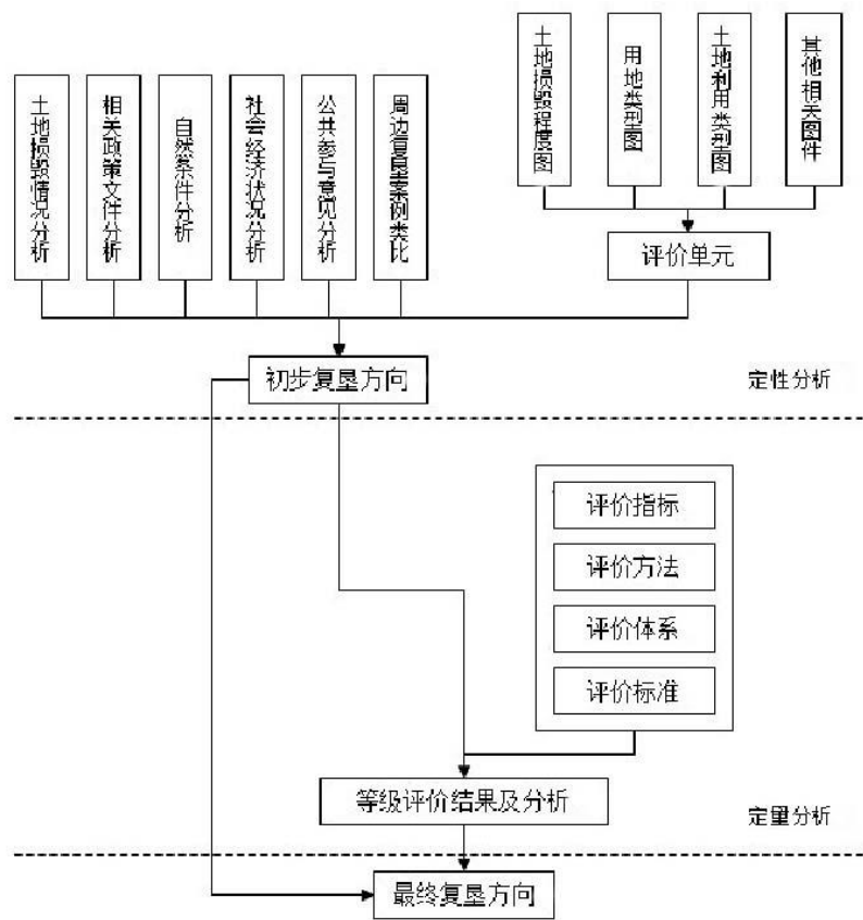
图4.1-1土地适宜性评价流程图
